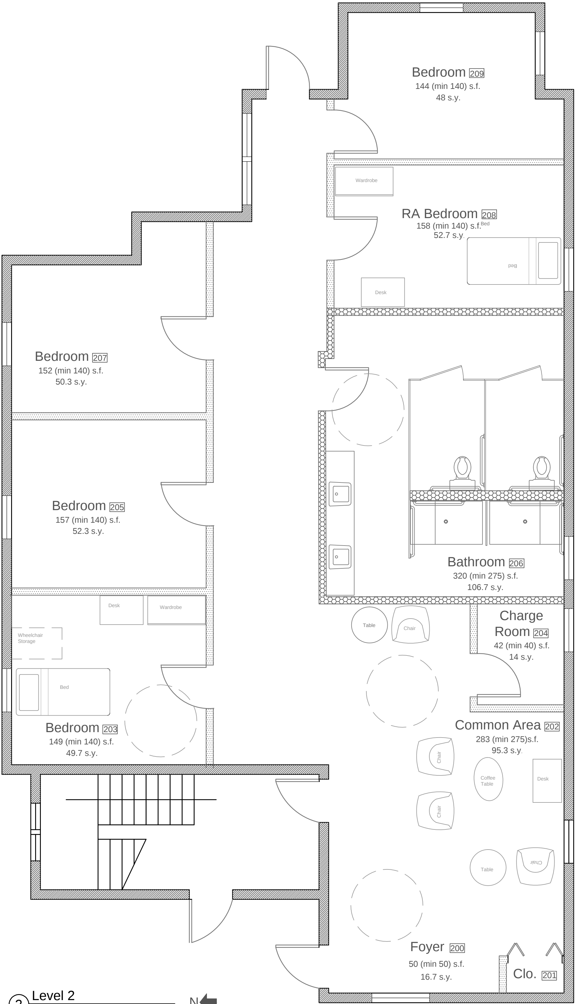
2 Level 2 Scale: 1/4"=1'-0"
